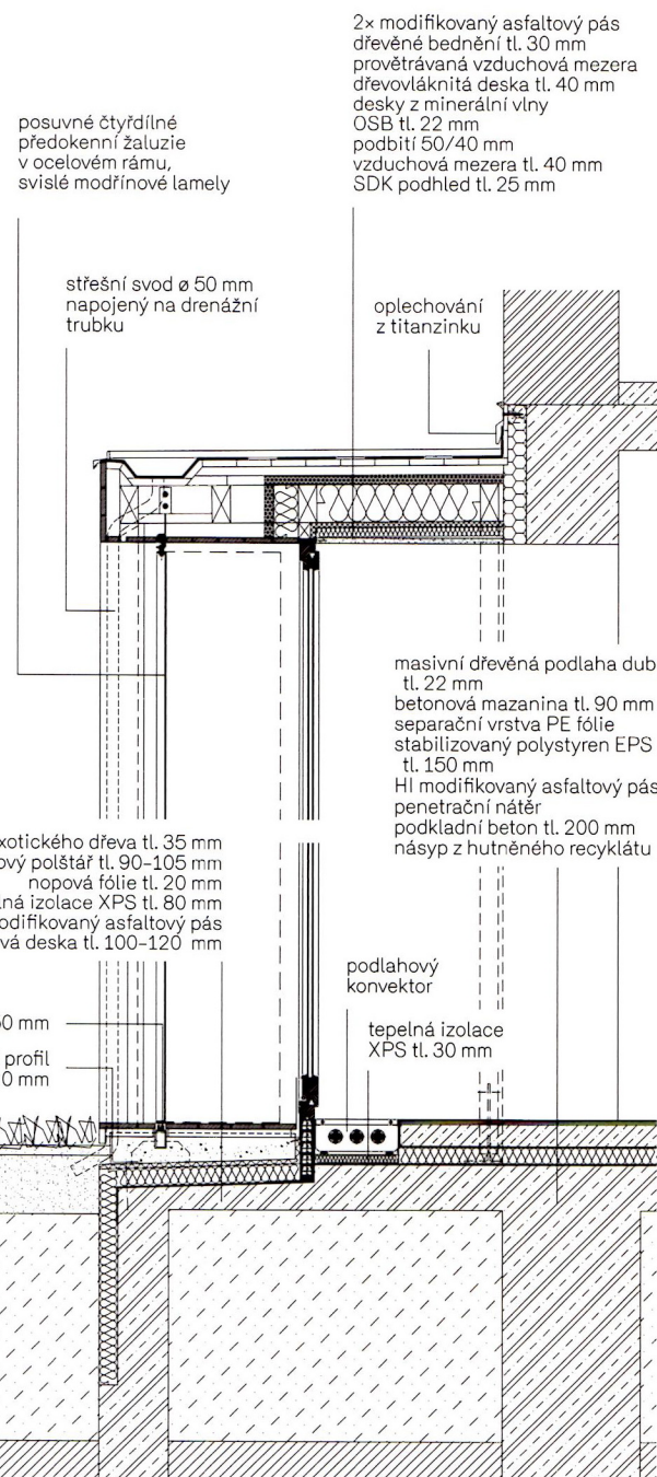
Detail konstrukce rizalitu jihovýchodní fasády
