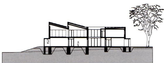
Řez A-A
